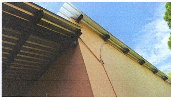
Foto 1: Sustrucción de lámina deteriorada por lámina troquelada.
